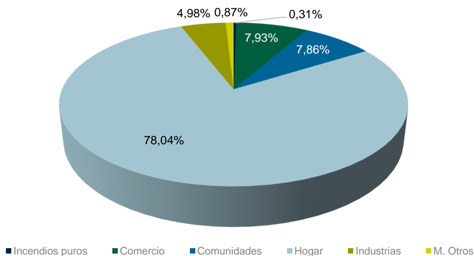
Ilustración 4: Distribución de los incendios por cobertura.
